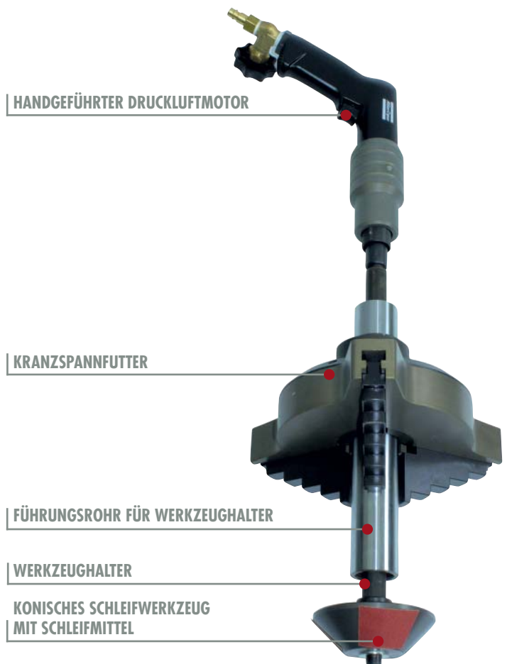
KVS 369/150 mit Kranzspannfutter
